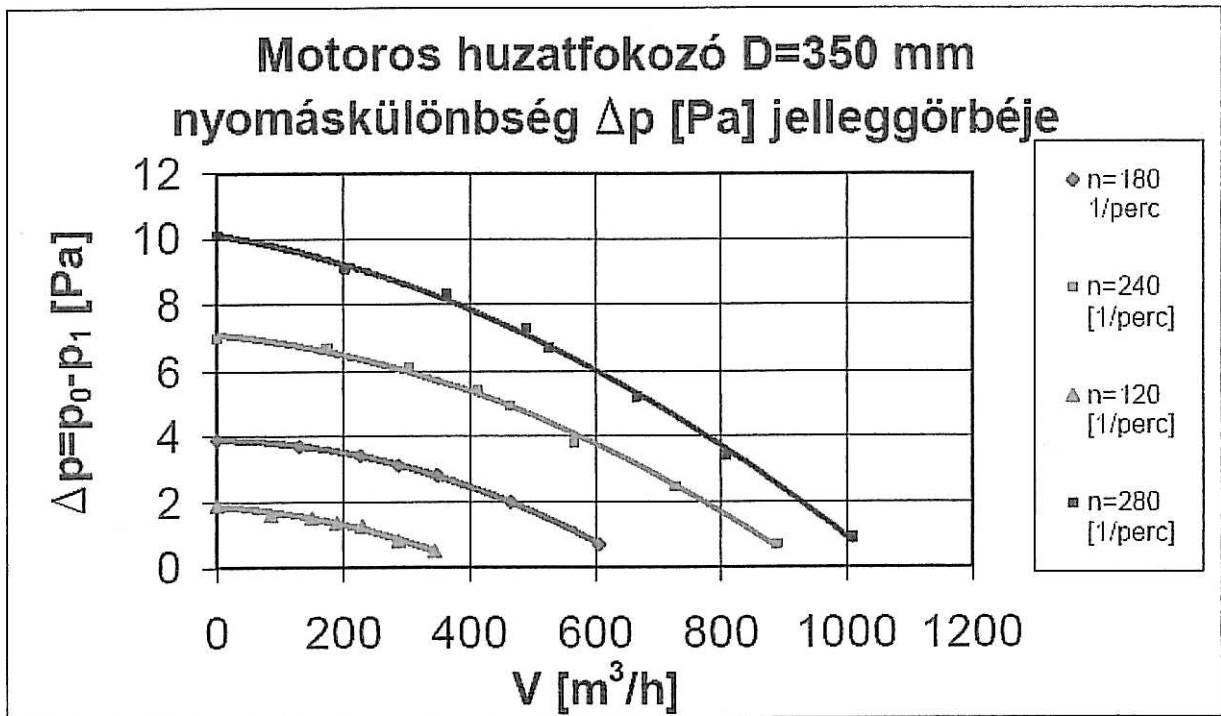
A huzatfokozó statikus nyomások különbsége, \Delta p a térfogatáram függvényében
