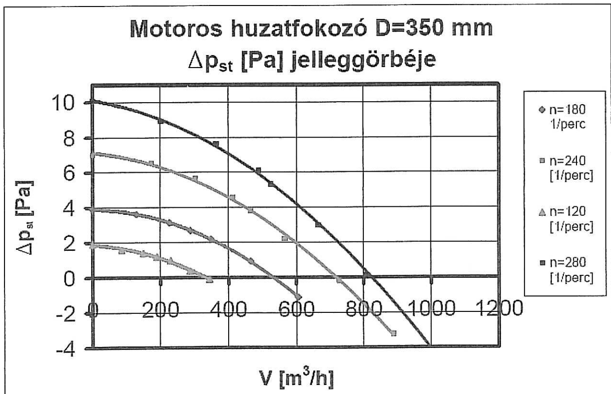
A huzatfokozó \Delta p_{st} = \Delta p - \frac{\rho}{2} \cdot v^2 nyomásnövekedés a térfogatáram függvényében
